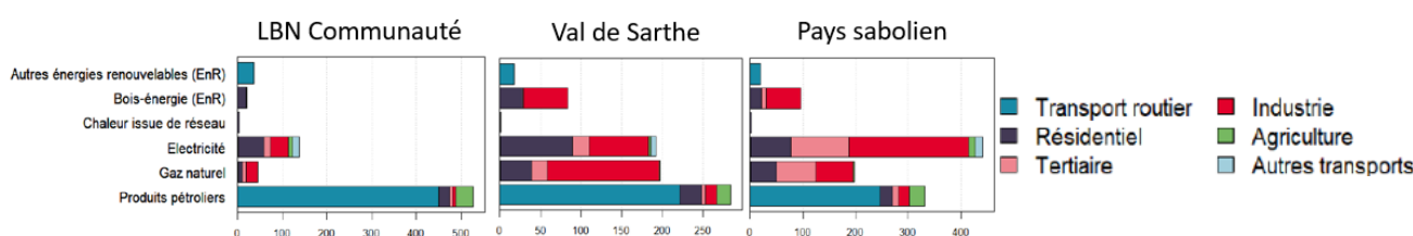
CONSOMMATION D'ÉNERGIE FINALE (GWh) PAR TYPE ET PAR SECTEUR SUR LES 3 CDC (2021) :
